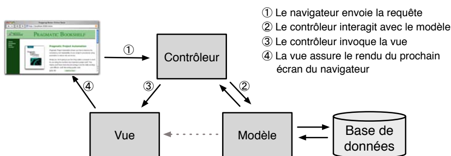
Figure 2-1 L'architecture modèle-vue-contrôleur
